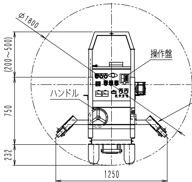
A 矢視図
